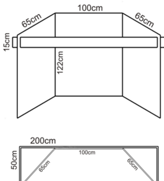
Figura 1 - Layout do estande modelo padrão. A testeira é opcional.
